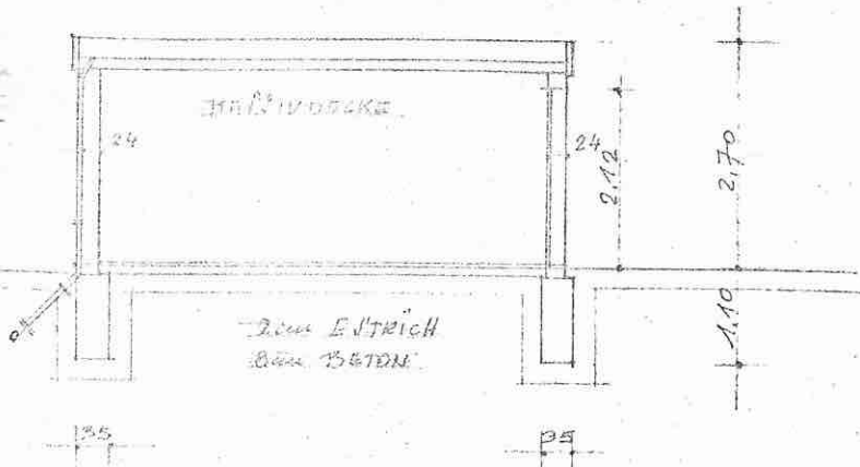
SCHNITT GARAGE
