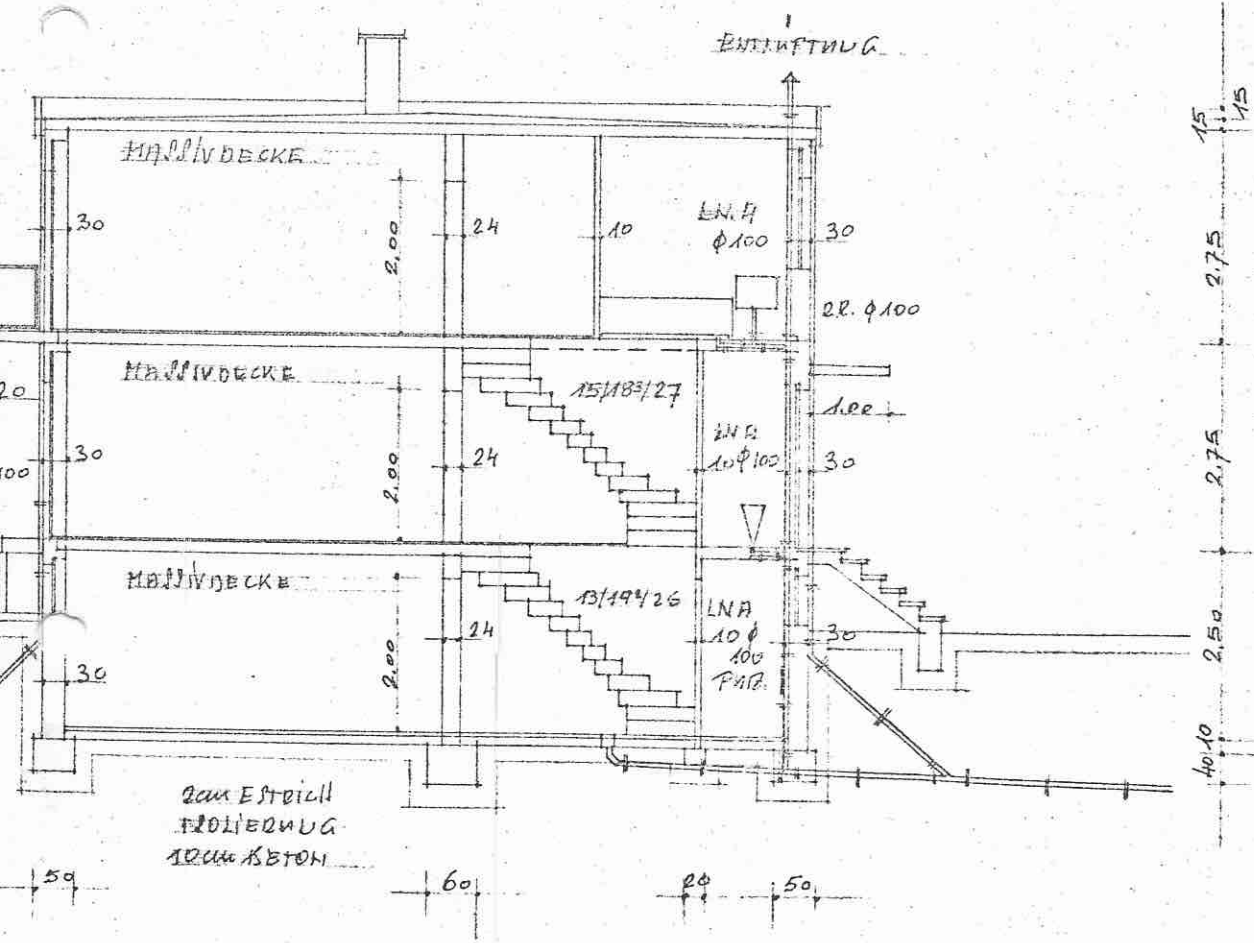
SCHNITT WOHNHAUS
