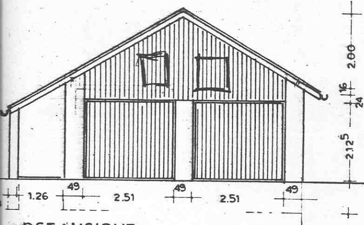
OSTANSICHT
