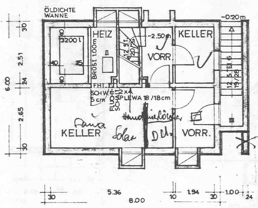
KELLERGESCHOSS
