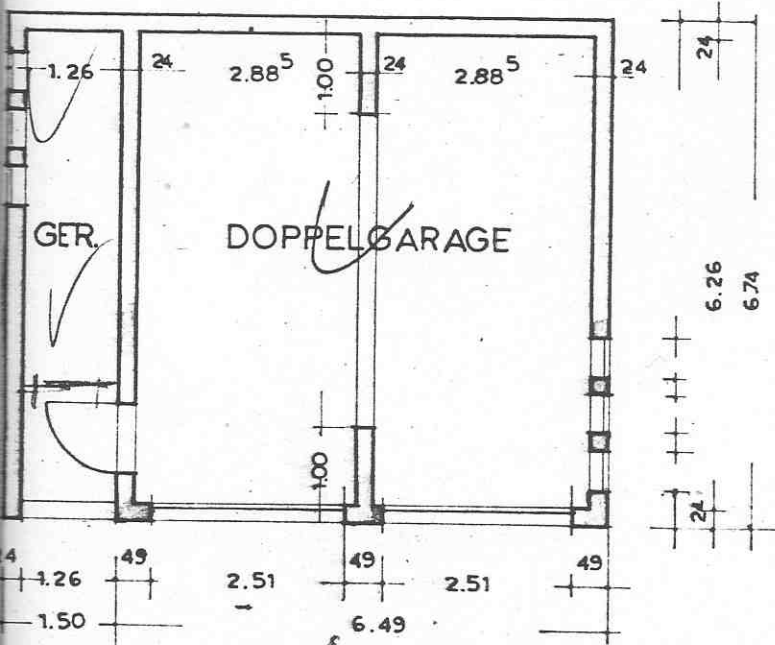
GRUNDRISS
