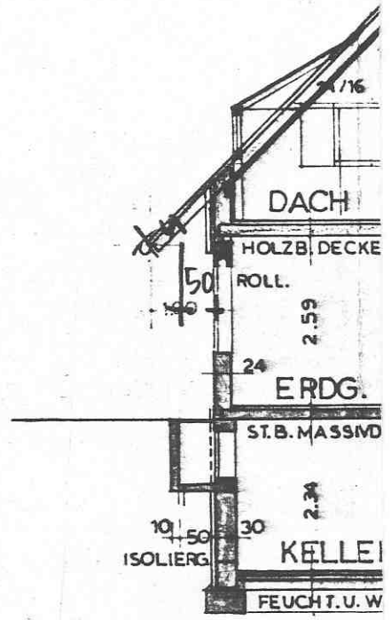
SCHNITT
