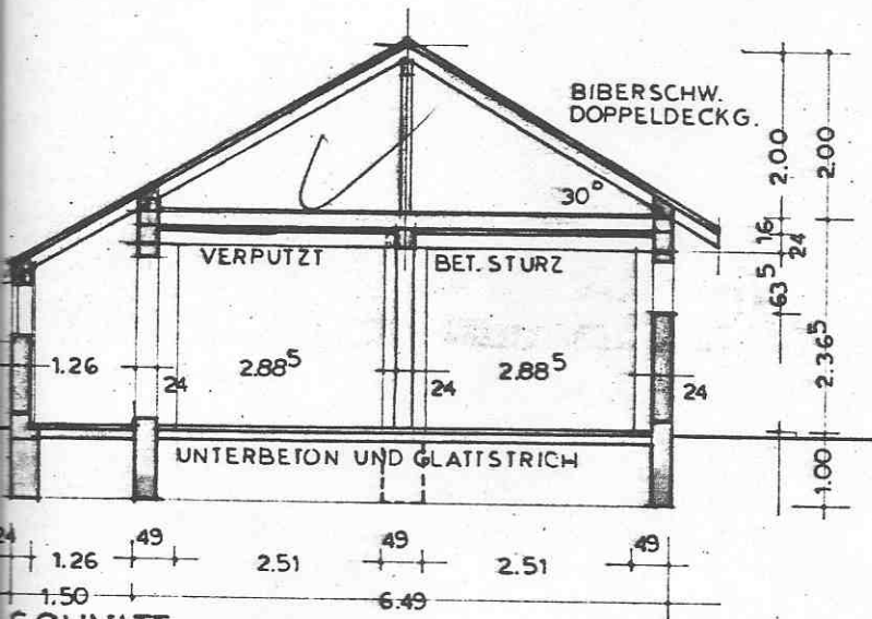
SCHNITT
