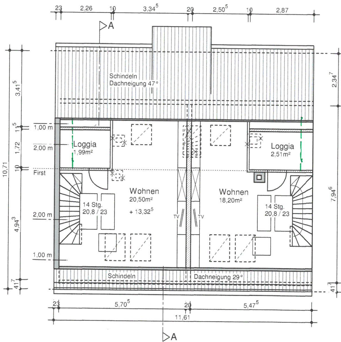
2. Dachgeschoss
