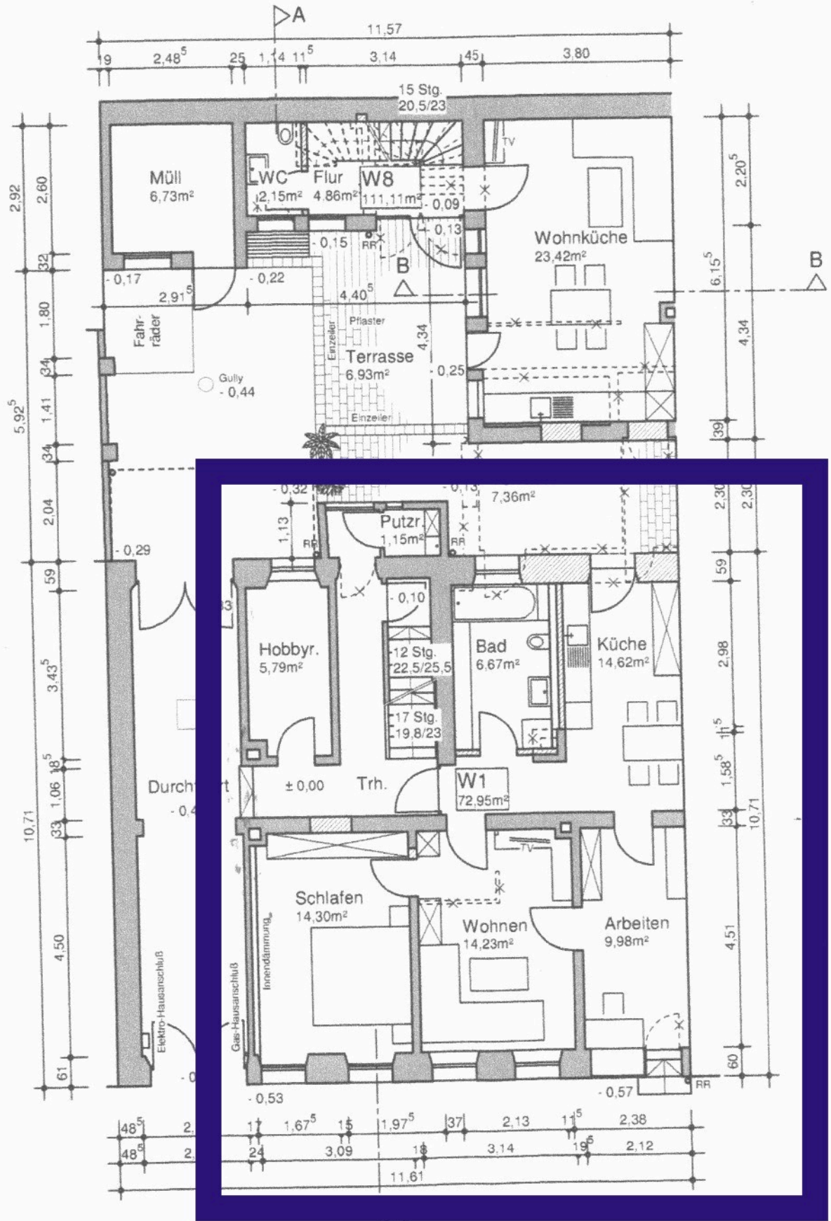
Erdgeschoss
