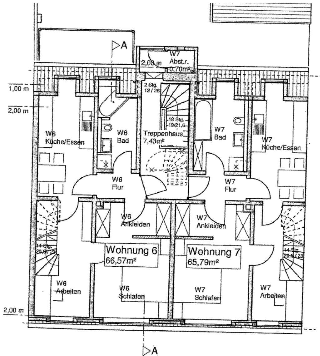
1. Dachgeschoss
